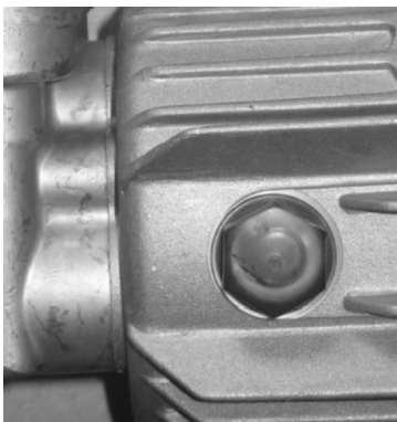
Εικόνα. Παράθυρα ελέγχου στάθμης λαδιού αντλίας.
